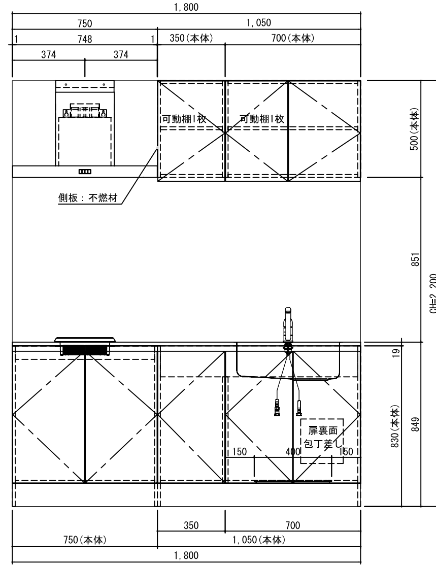
正面図
